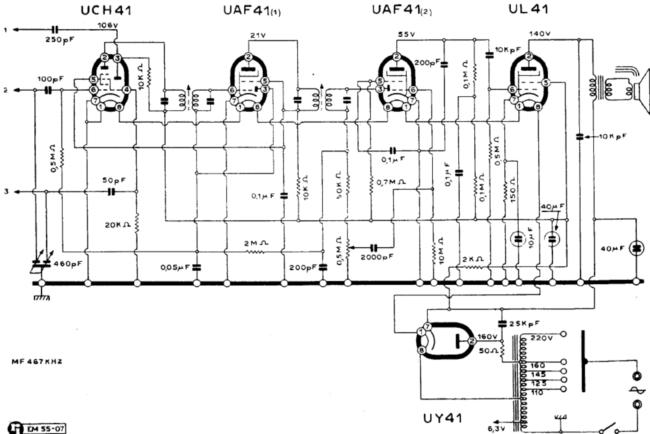
ELECTA RADIO - Mod. 520A
